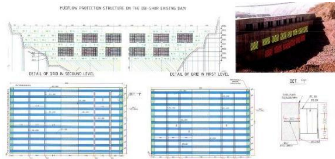
Расми 9. Навсоии оббанди мавҷудаи Обишӯр
