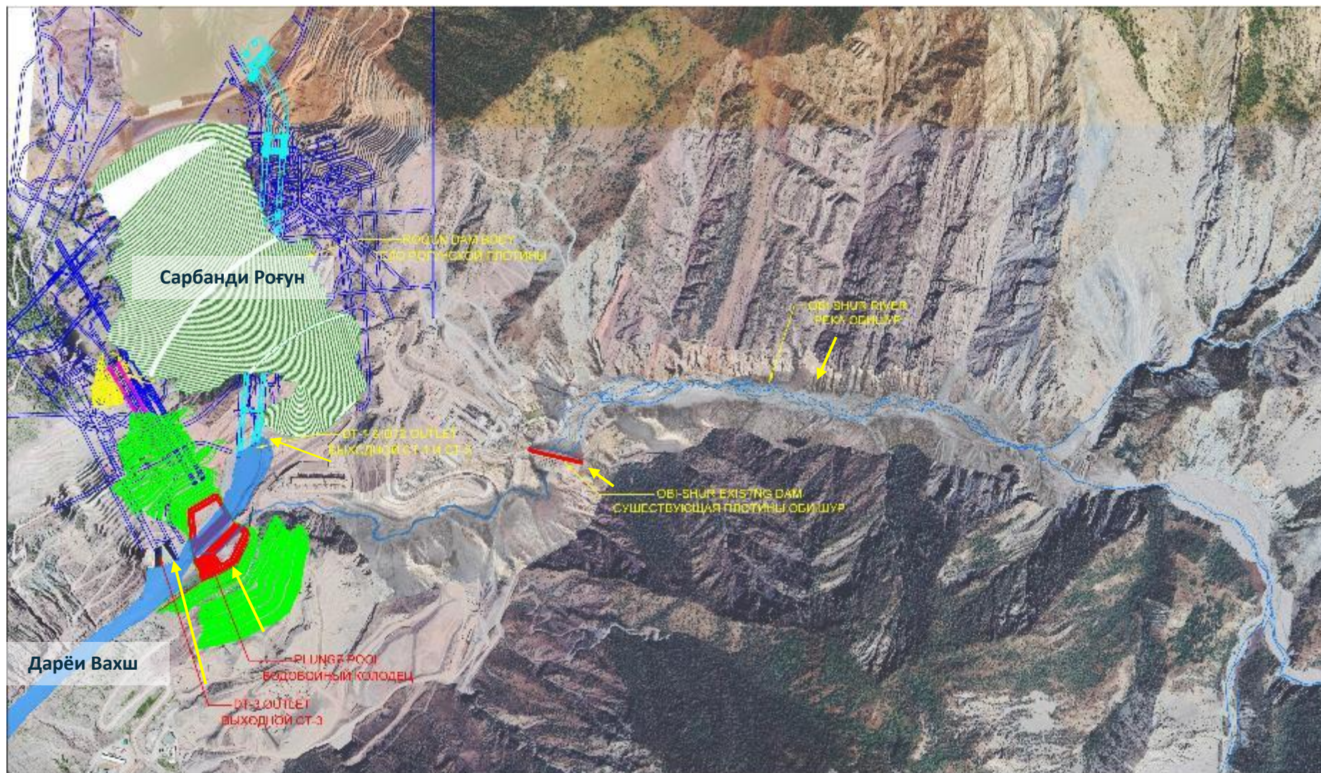
Расми 1. Нақшаи умумии ҷойгиршавии оббанди Обишӯр ва иншооти поёнобии НБО-и Роғун
